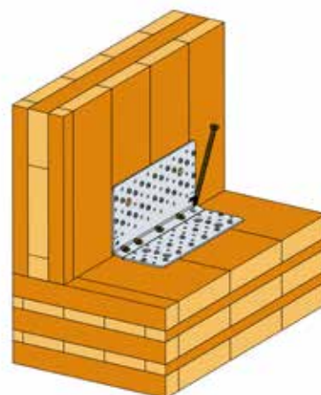
Hout op hout
