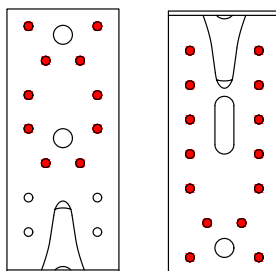
Bevestiging op houten ondergrond
