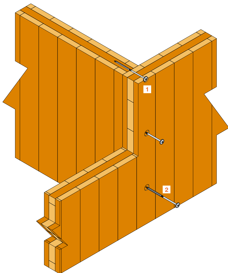
1 ESCR - Constructiehoutschroef platte kop
