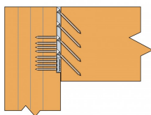
Fixation sur poteau (montage invisible avec lamage)
