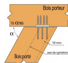
Assemblage en angle - Vue de dessus
