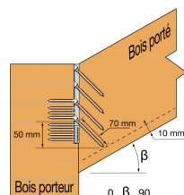
Assemblage en pente - Pente positive uniquement
