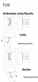
Schuine verbinding op kolom
